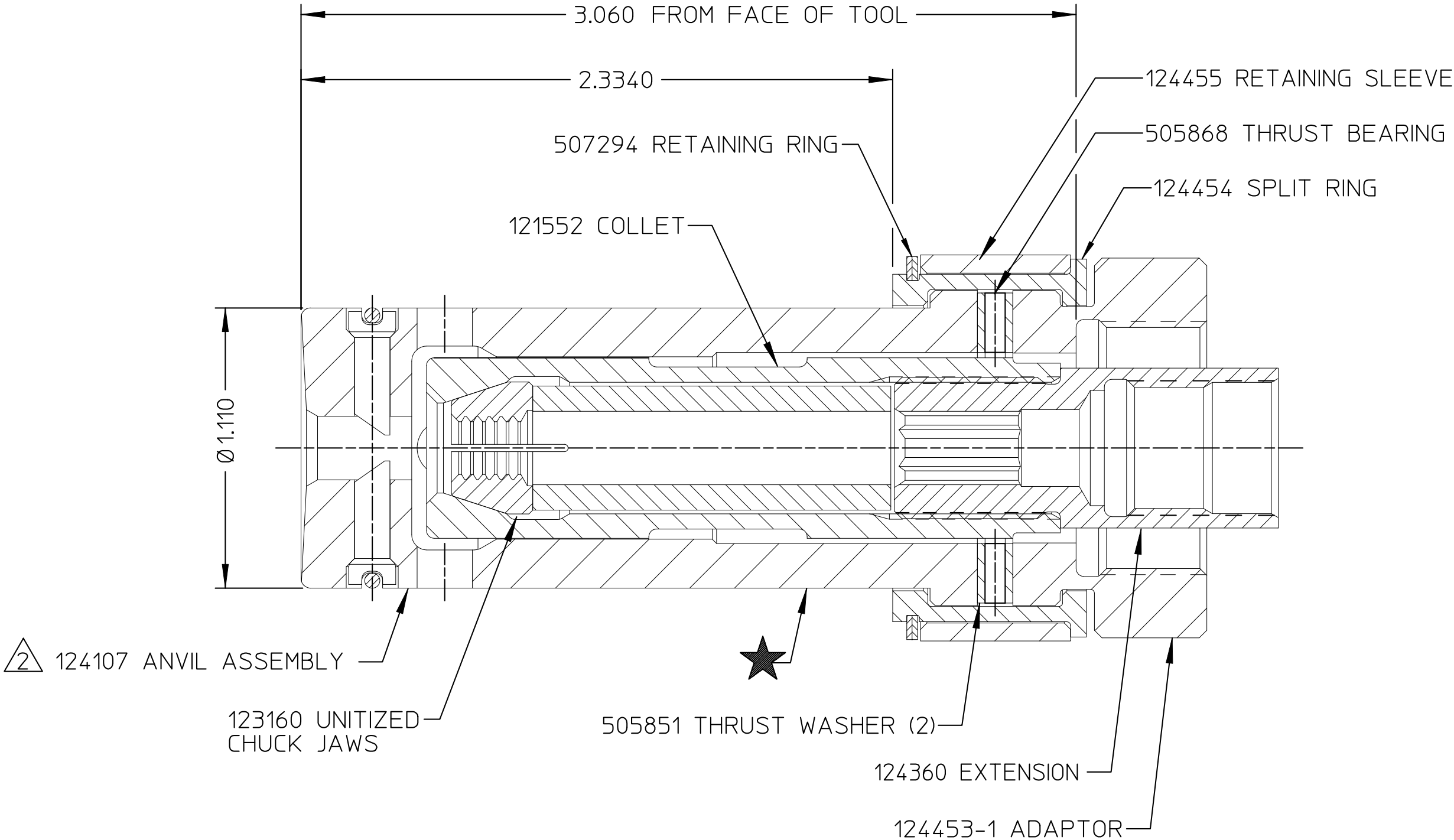
SECTION A-A
