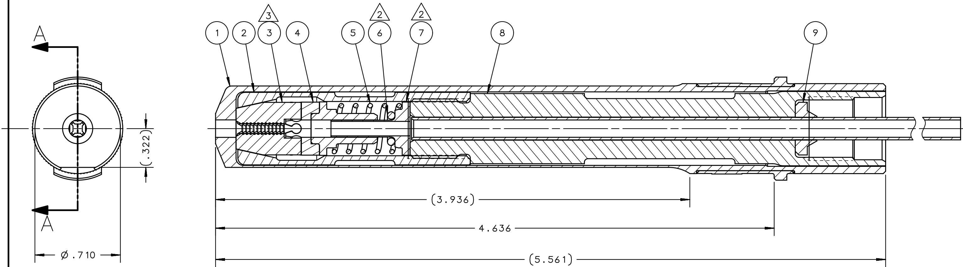
SECTION A-A
