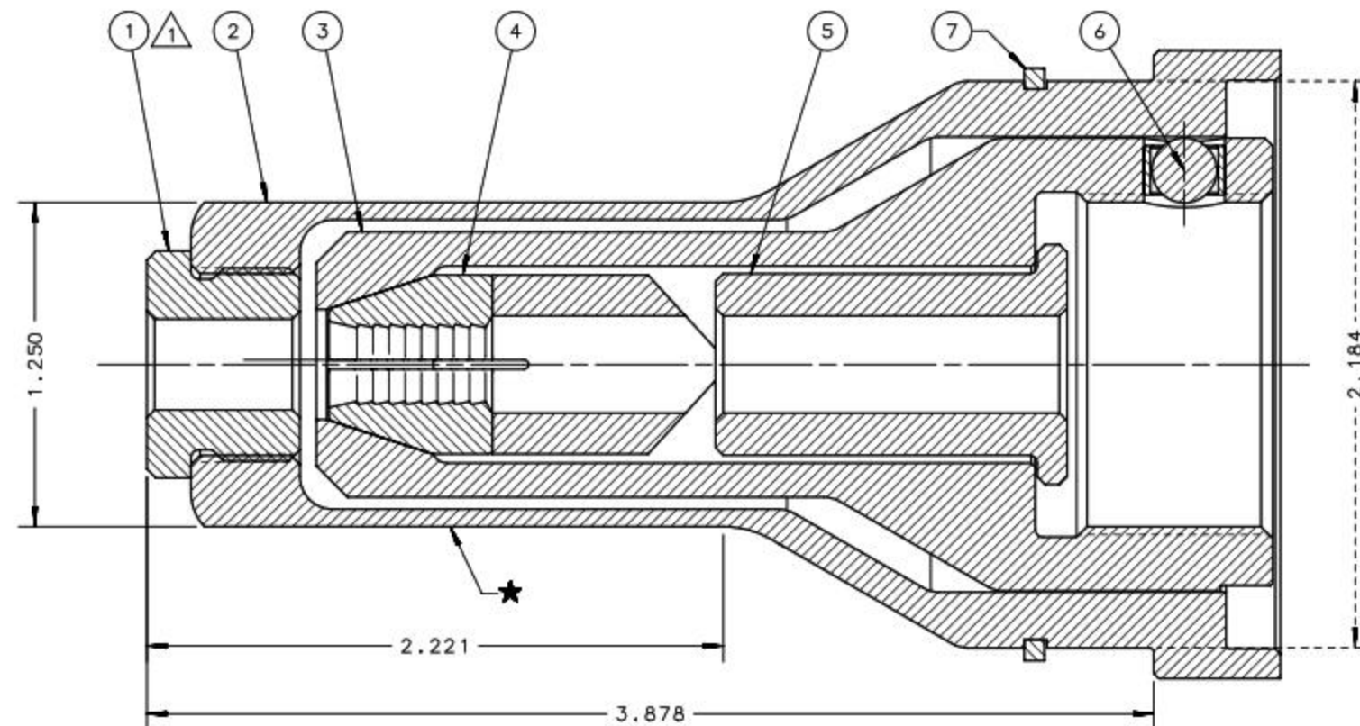
SECTION A-A
