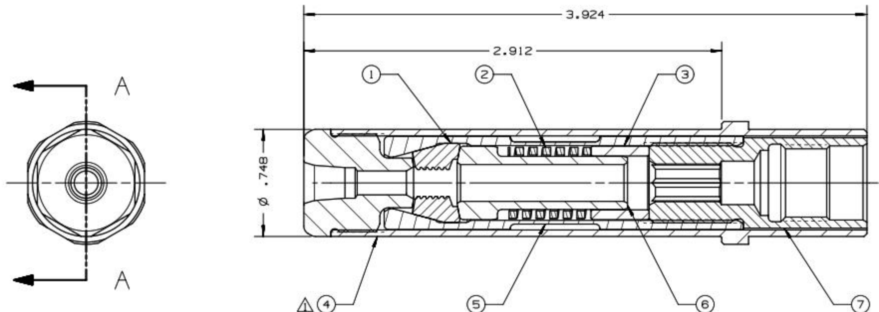
SECTION A-A
