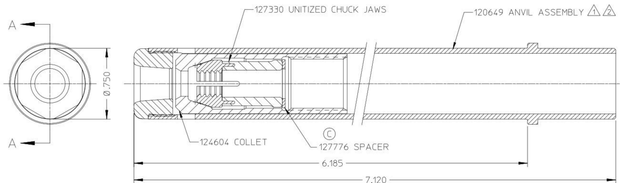
SECTION A-A
