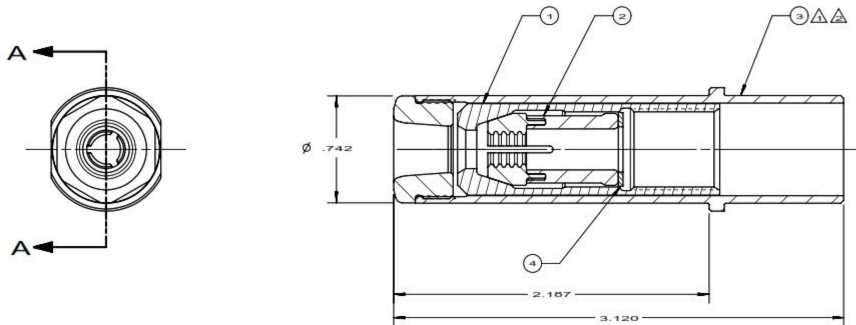
SECTION A-A
