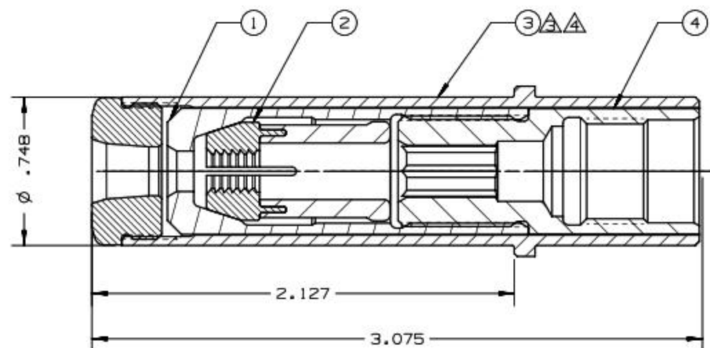
SECTION A-A
