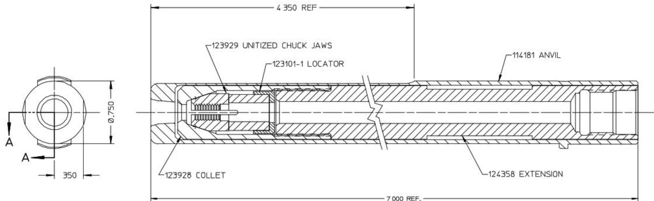
SECTION A-A
