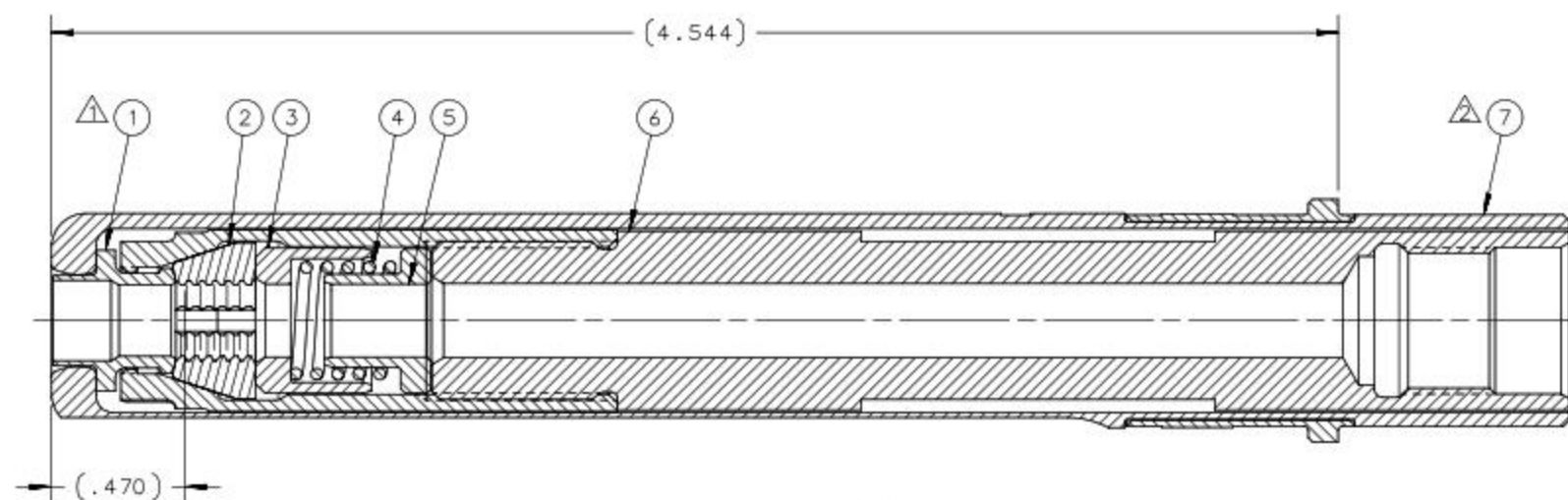
SECTION A-A
