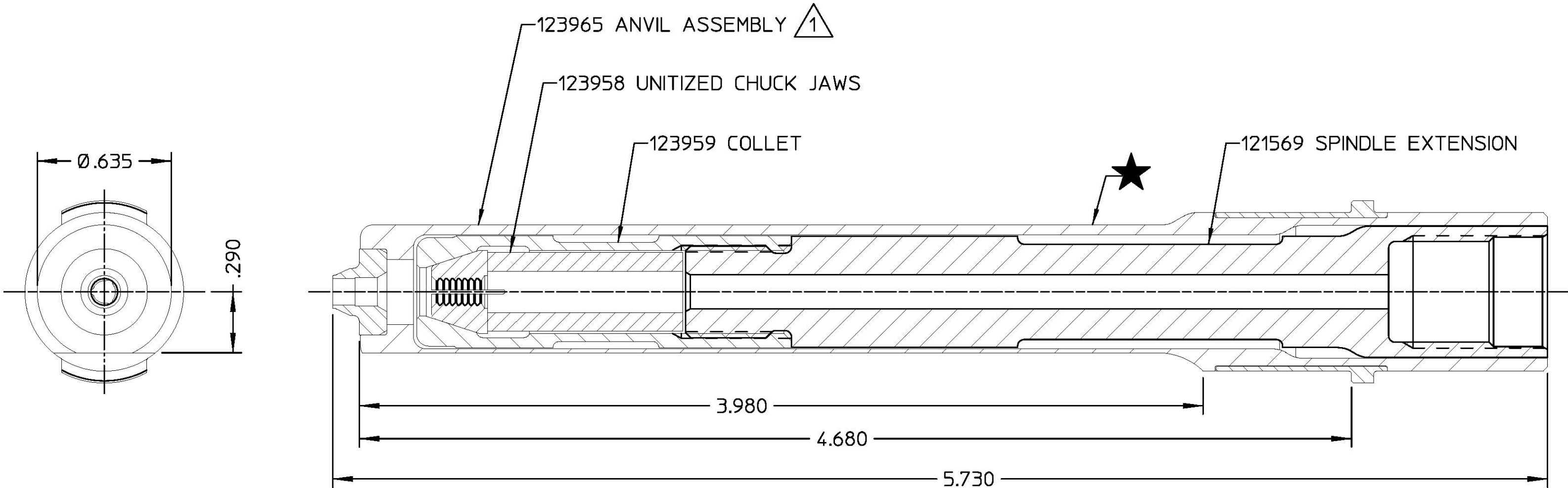
SECTION A-A
