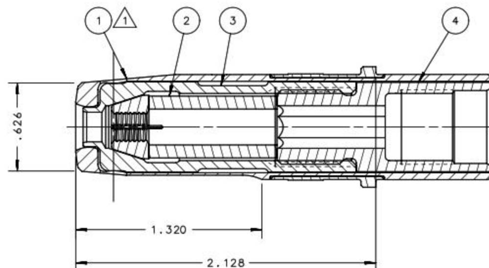
SECTION A-A
