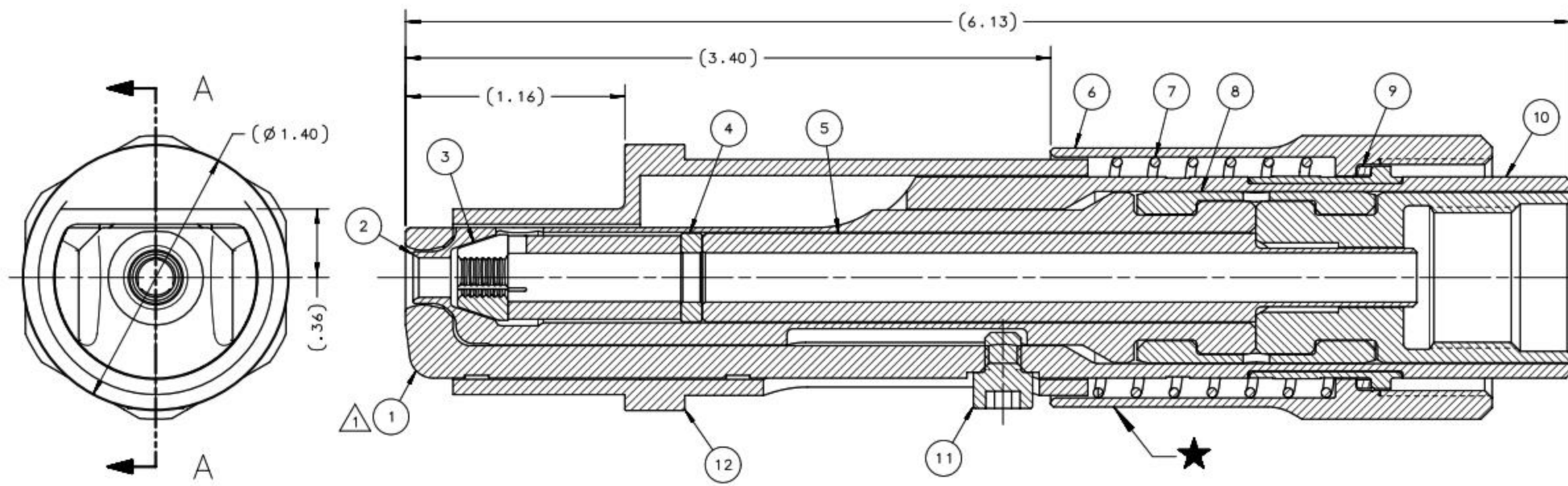
SECTION A-A
