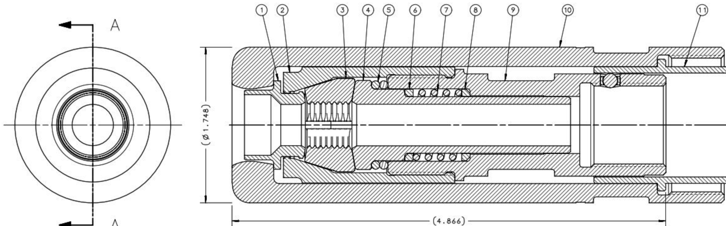
SECTION A-A
