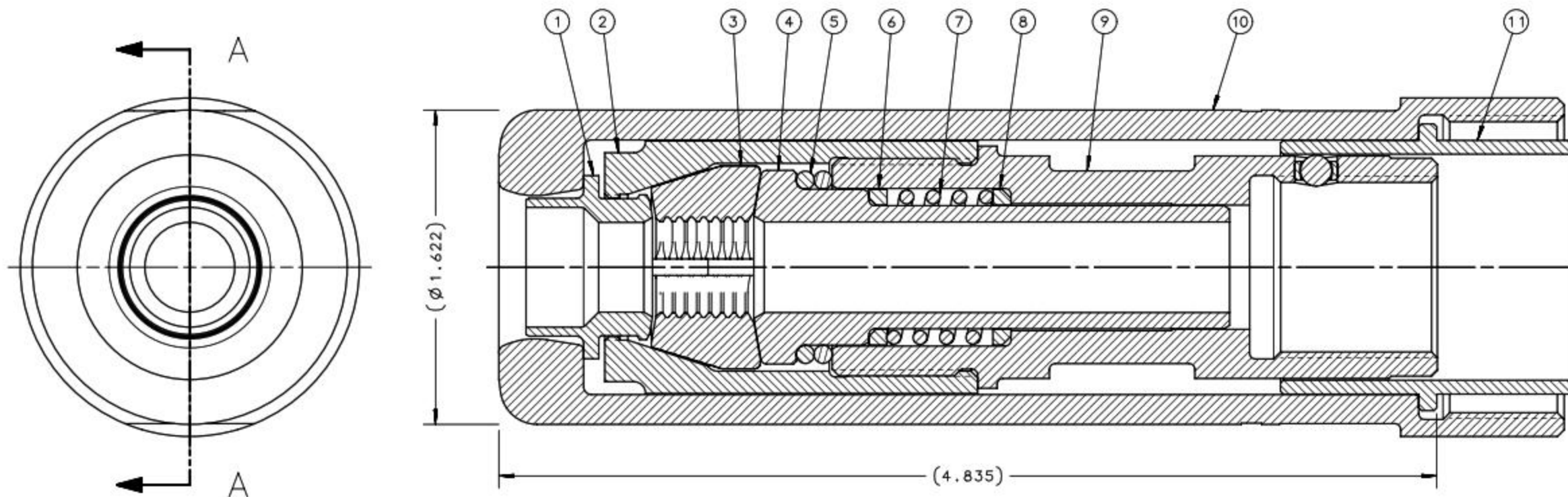
SECTION A-A
