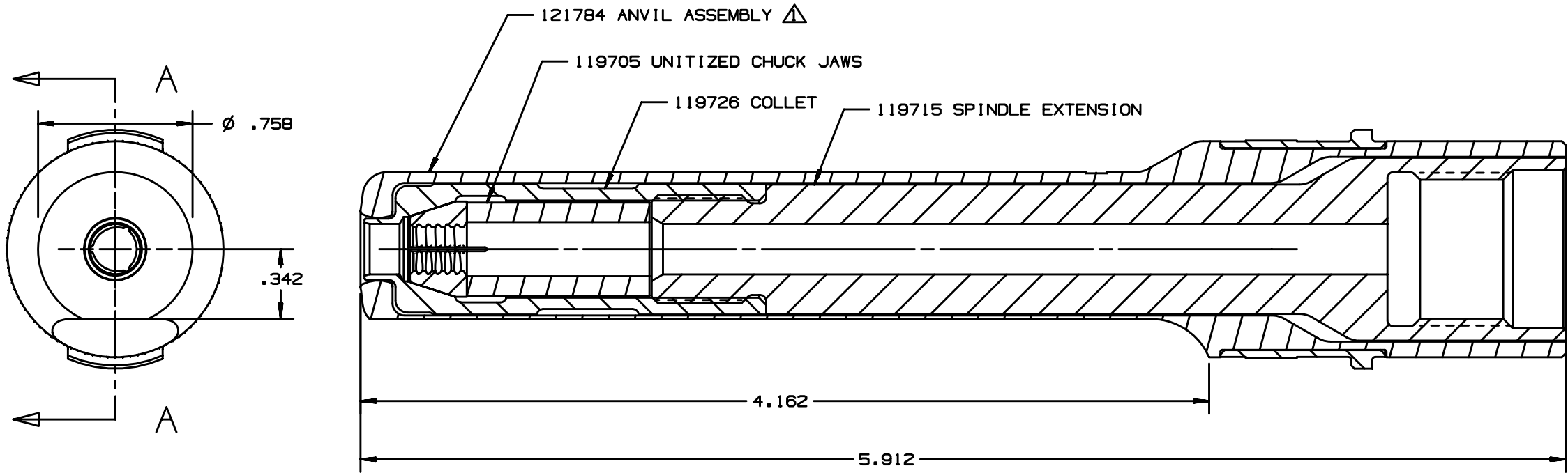
SECTION A-A
