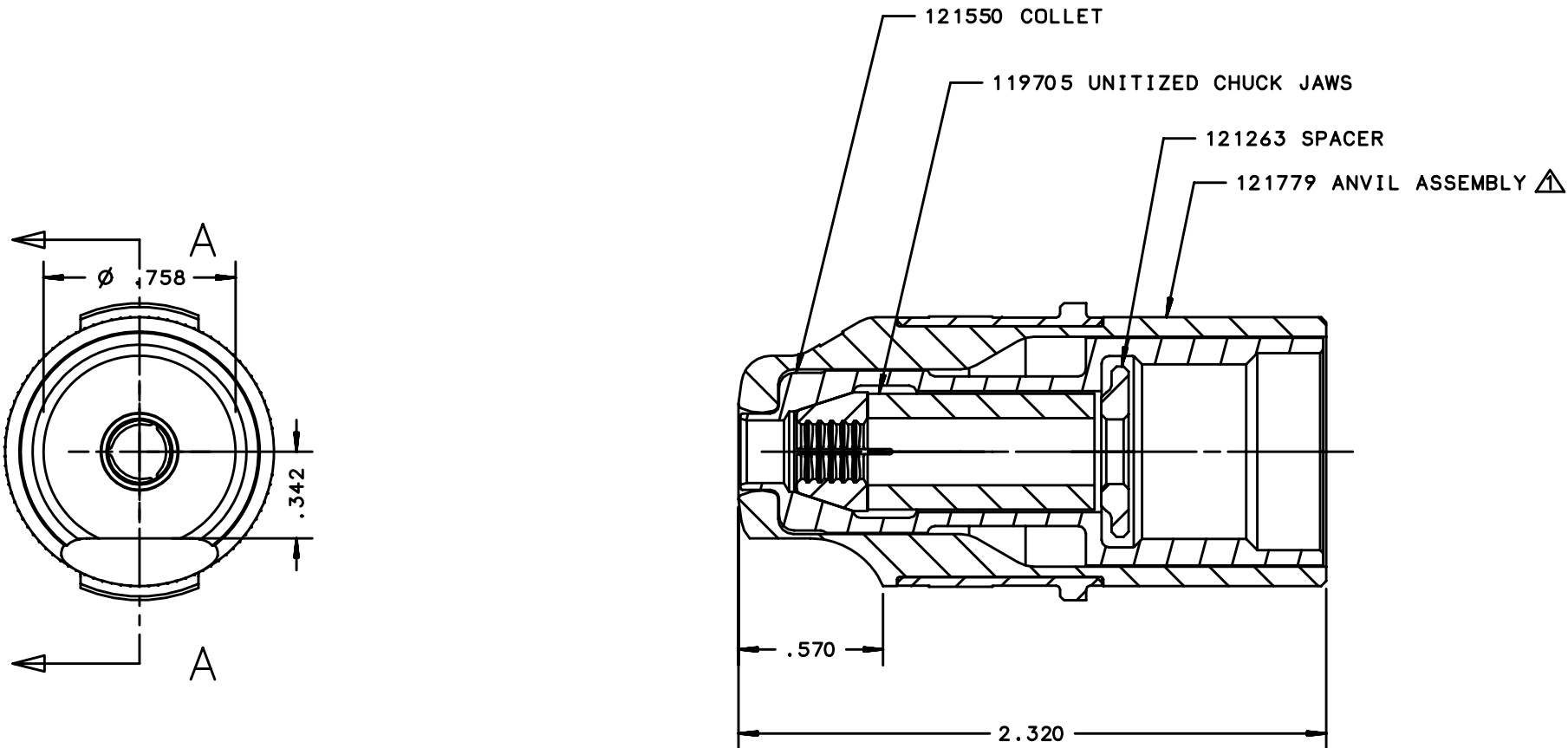
SECTION A-A
