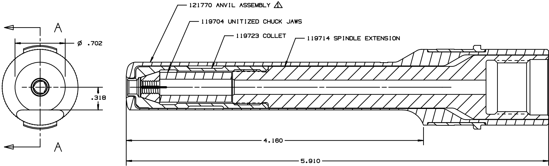
SECTION A-A
