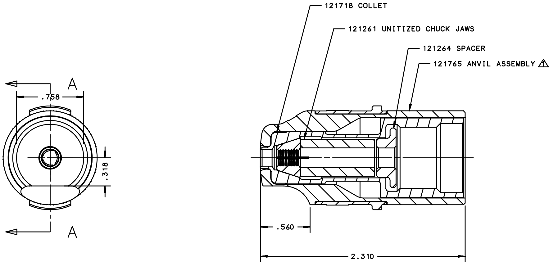
SECTION A-A
