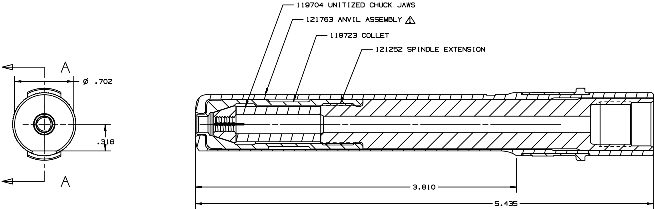
SECTION A-A
