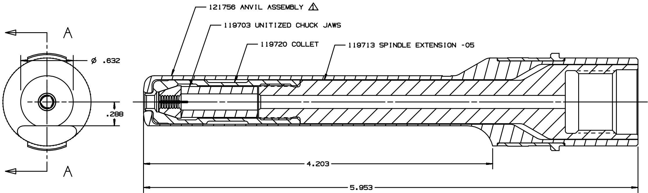
SECTION A-A
