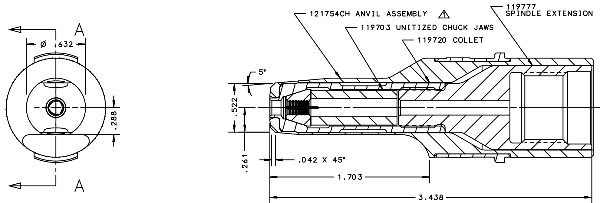
SECTION A-A
