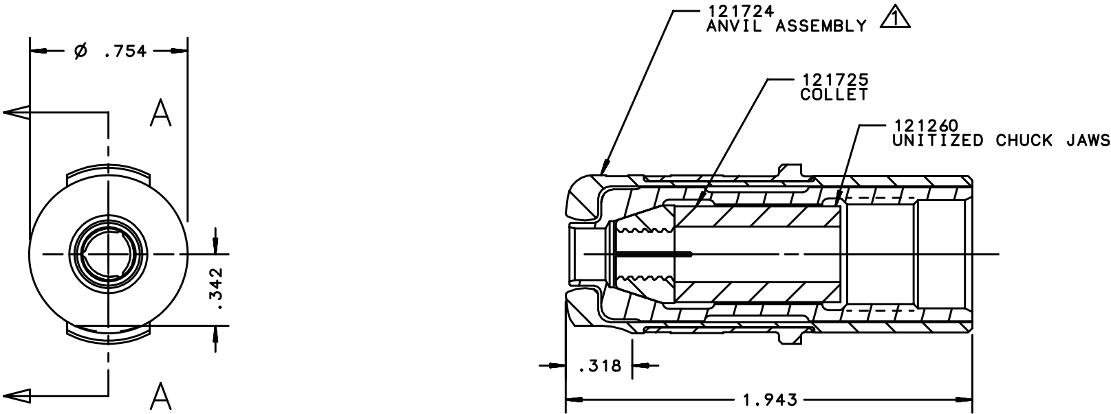
SECTION A-A
