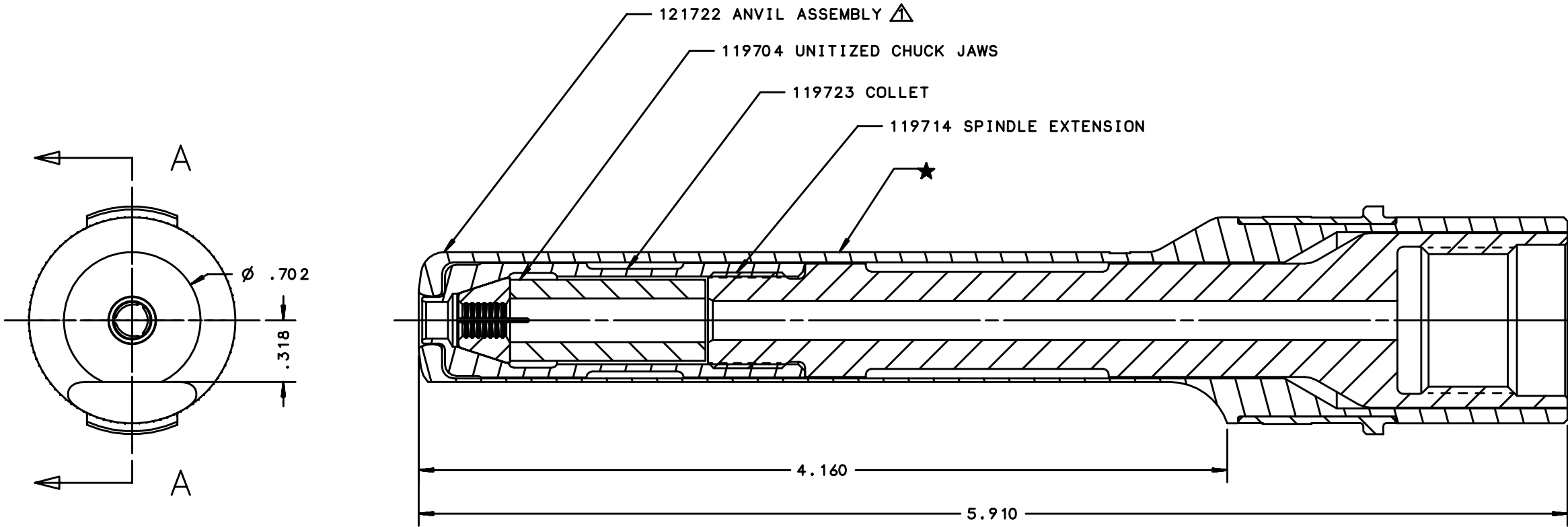
SECTION A-A
