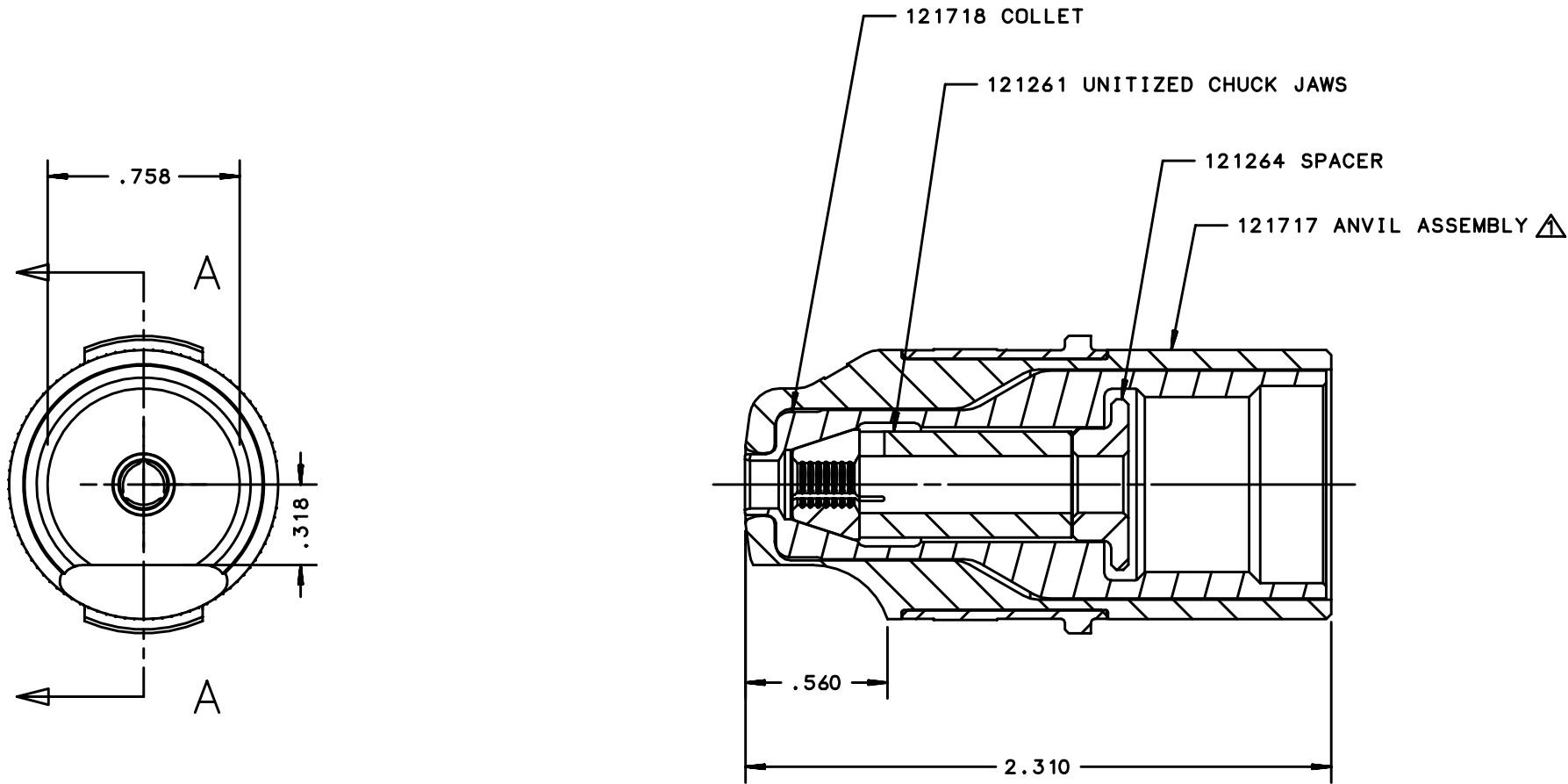
SECTION A-A
