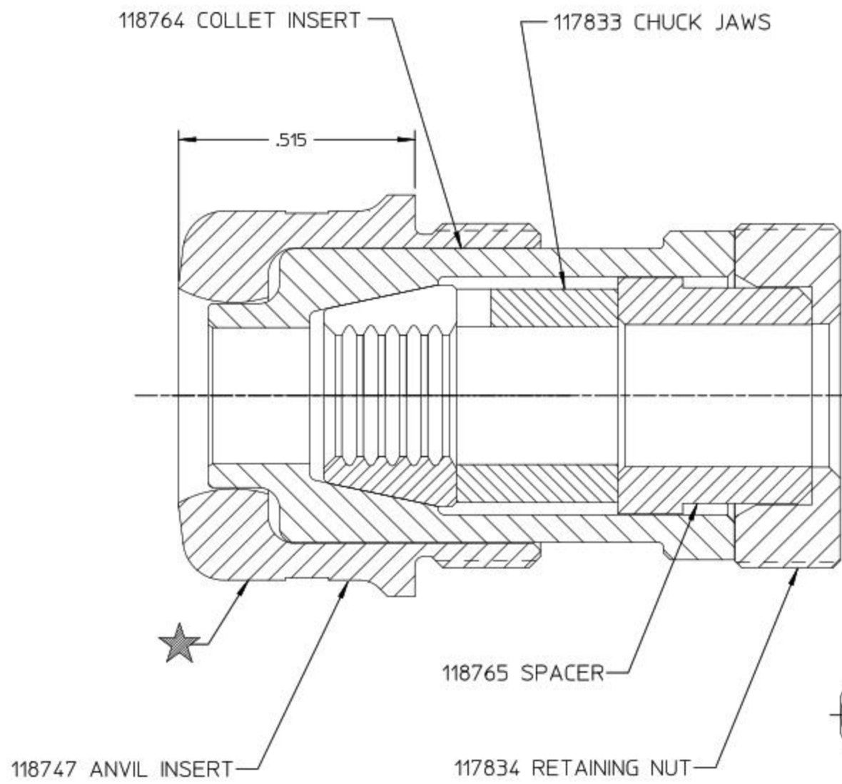
SECTION A-A
