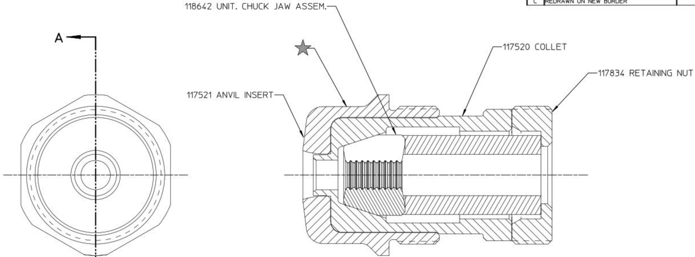
SECTION A-A
