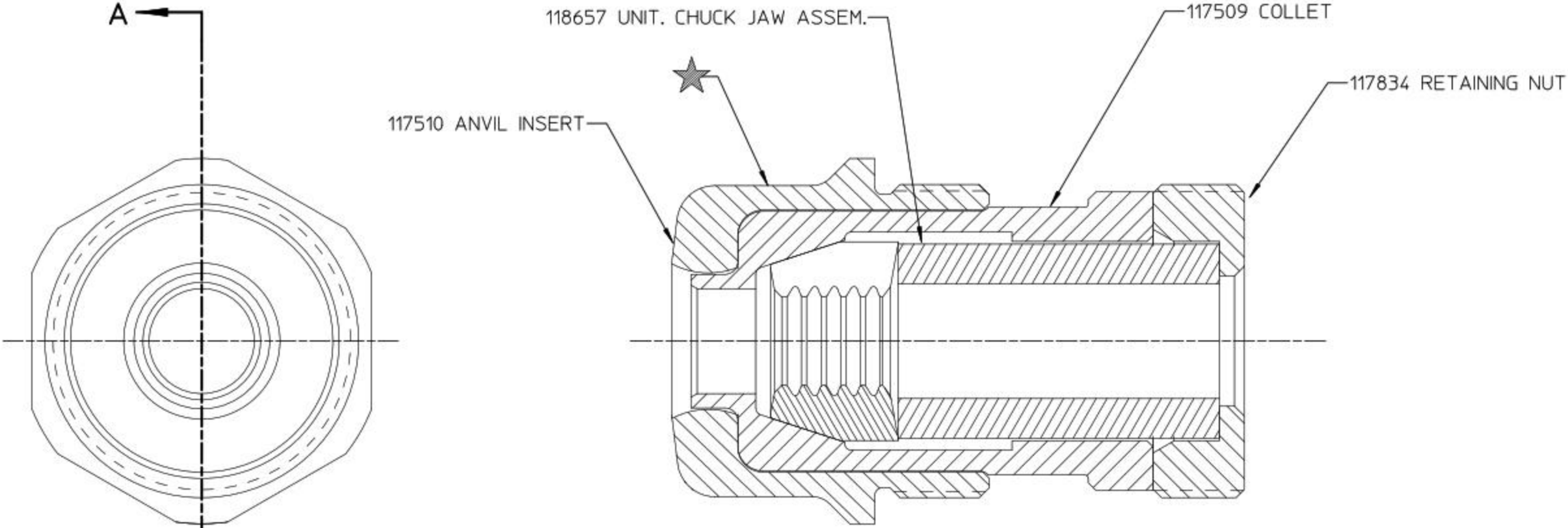
SECTION A-A
