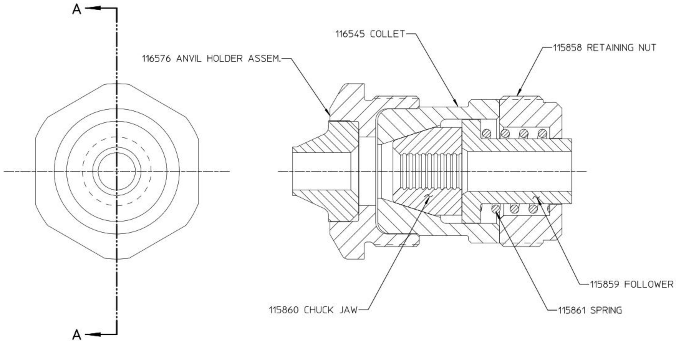
SECTION A-A
