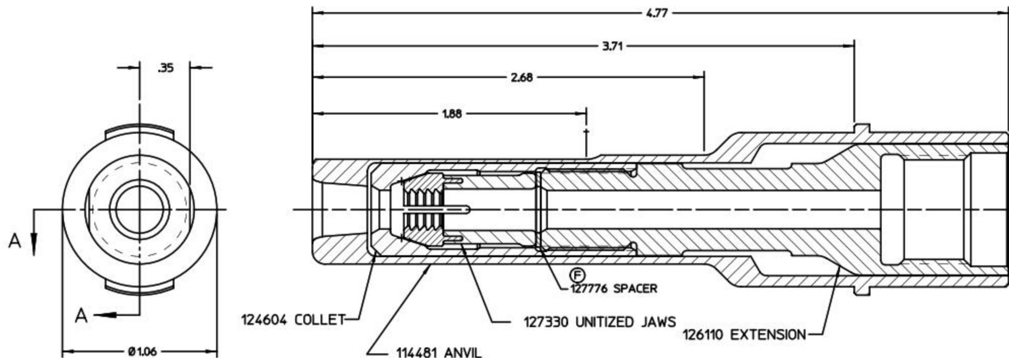
SECTION A-A
