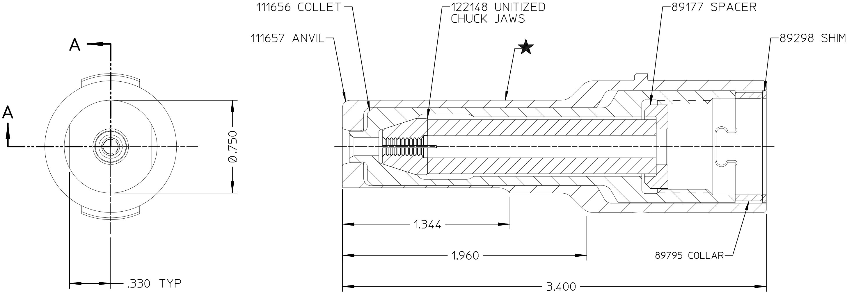
SECTION A-A
