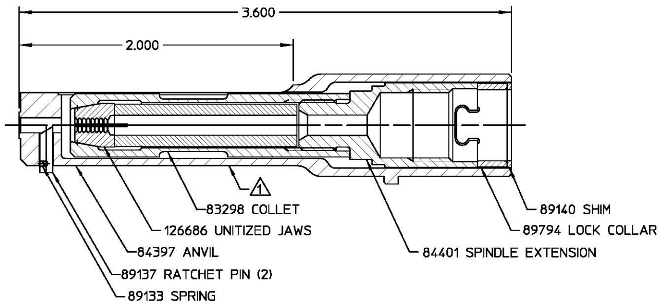
SECTION A-A
